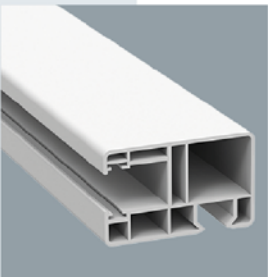
39mm Pvc Yan Ray 39 mm Pvc Side Rail Profile 39 mm ПВЦ странична водилка
