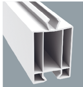
Öteleme Profili Pushing Profile PVC (44mm) ПВЦ дистанцер 44 mm
