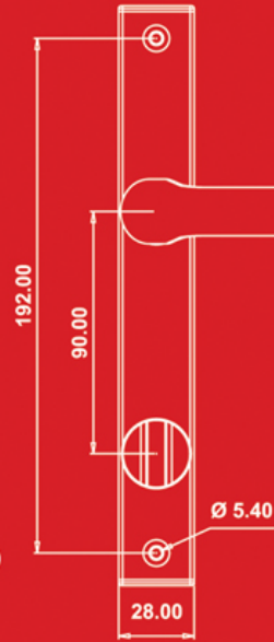
3010-72 Ares WC Kapı Kolu (Dar Ayna) Ares Door Handle – WC Type
