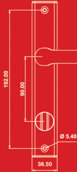
3010-62 Ares WC Kapı Kolu (Yaylı) Ares Door Handle - WC Type
