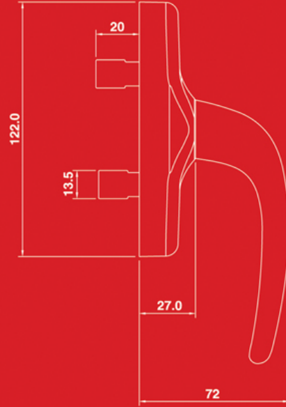
1822 Eksenel Kol (Çift maça) Cremone Handle
